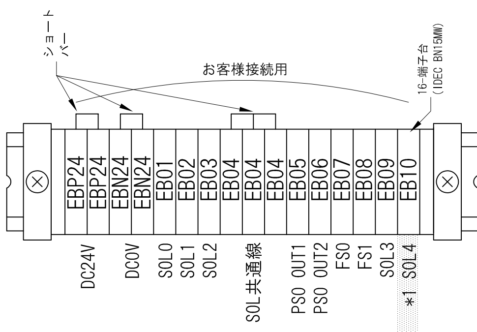
端子台結線図
